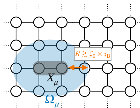
図：開放量子多体系の基礎方程式の導出のアイデア。リープ・ロビンソン限界を用いることで、多体系で重要となる局所性をもつ量子マスター方程式が得られる。arXiv:2404.14067 より転載。
